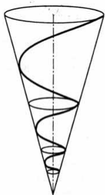
Figure 2. Une spirale logarithmique sur un cône.
